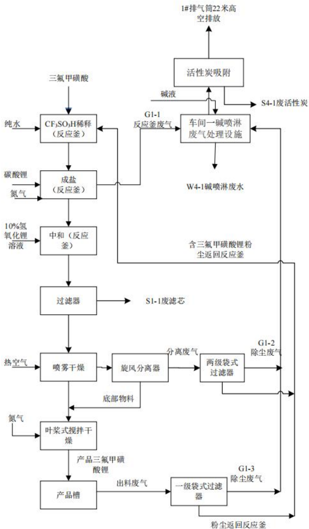
图 4-4 三氟甲磺酸下游产品项目生产工艺流程简
